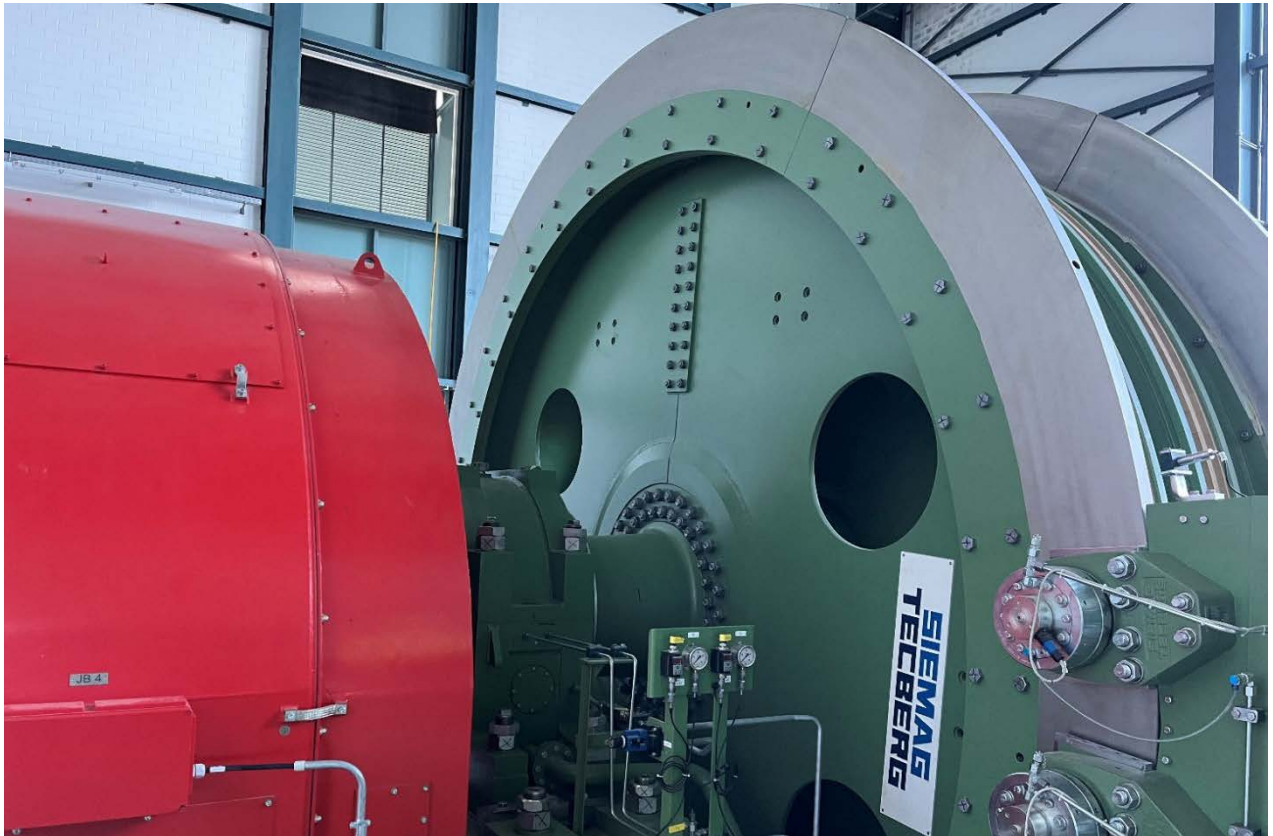
Abbildung 3: Schachtförderanlage Nord, Stand Herbst 2022
