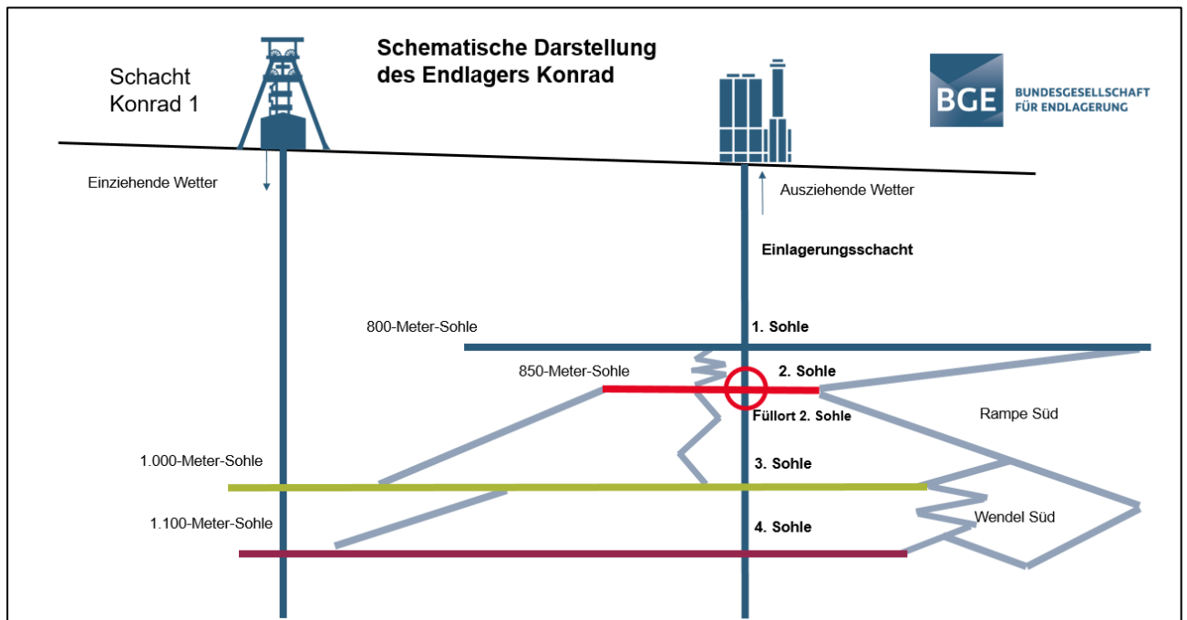
Abbildung 1: Schematische Darstellung des Endlagers Konrad
