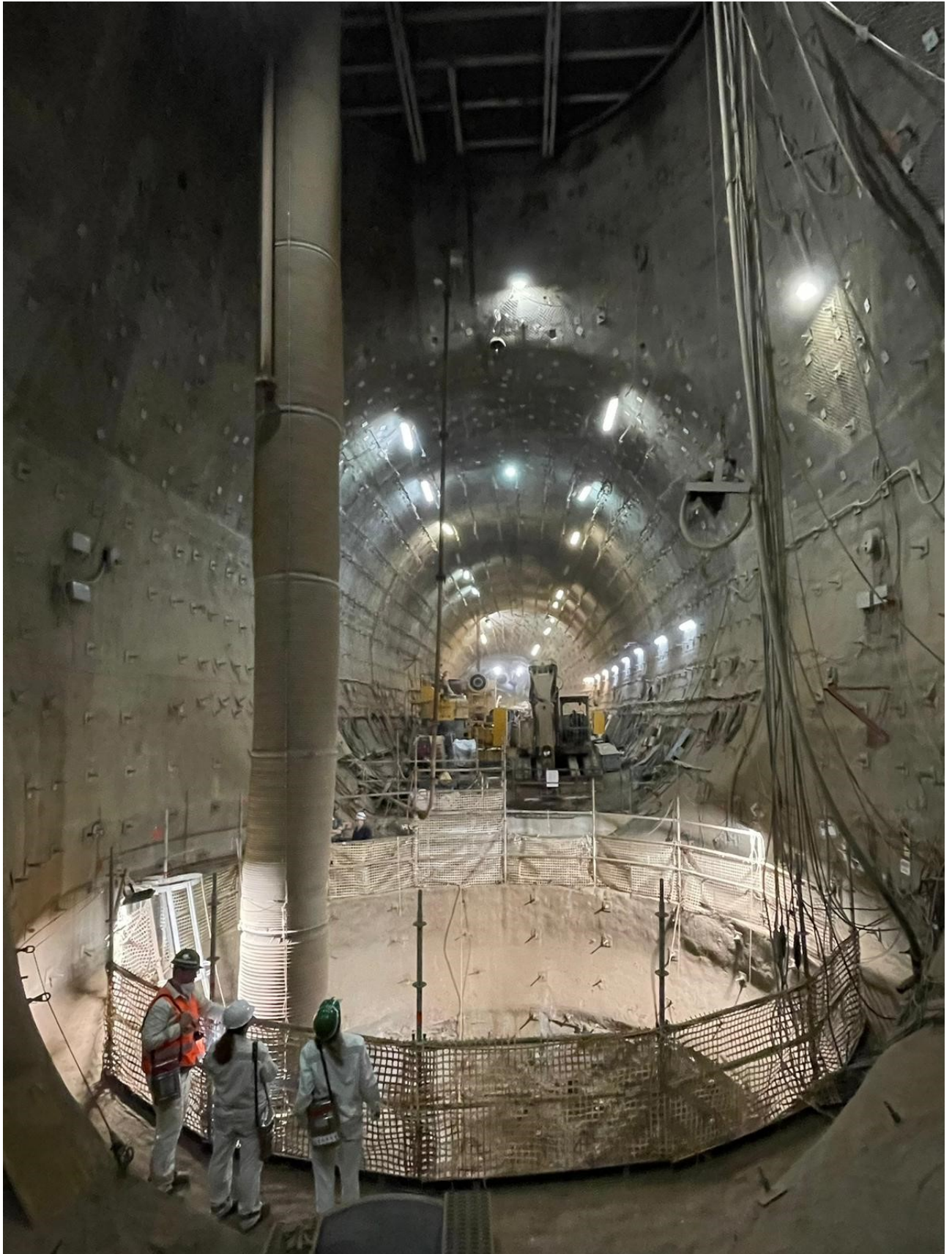
Abbildung 7: Einbringen der Innenschale am Füllort 2. Sohle
